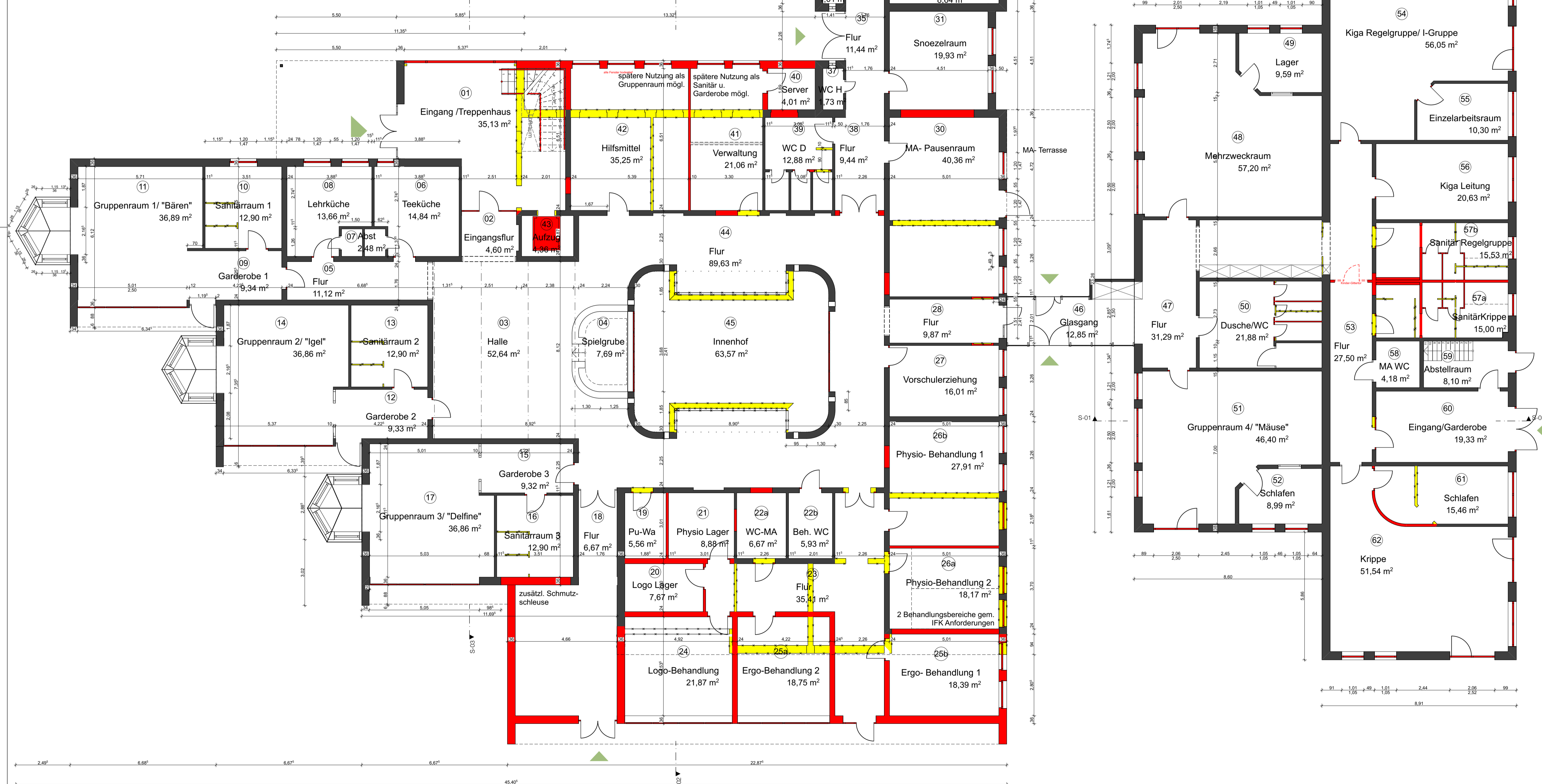
Vorentwurf Grundriss EG
