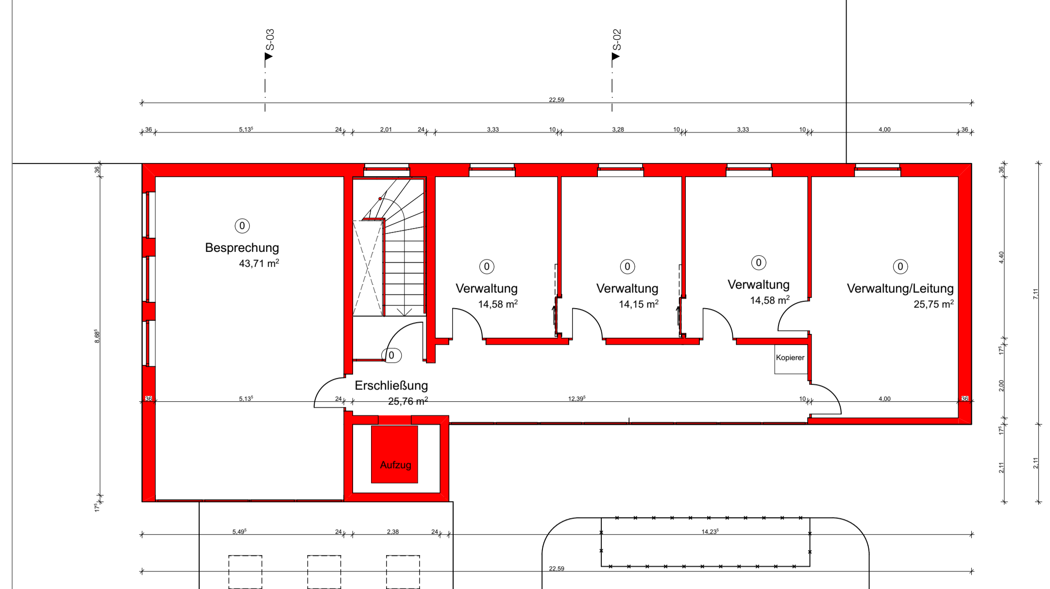
Vorentwurf Grundriss OG (Verwaltungsaufbau)
